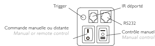
Panneau de contrôle Control panel
